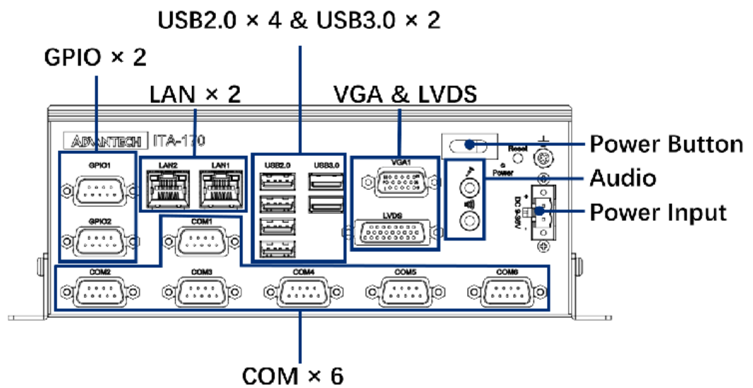
ITA-170 前视图
