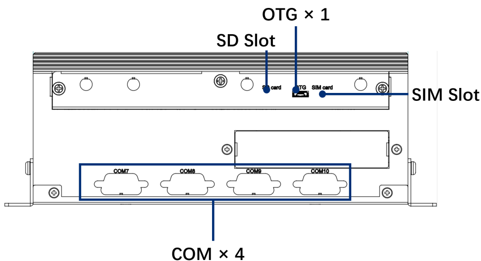
ITA-170 后视图
