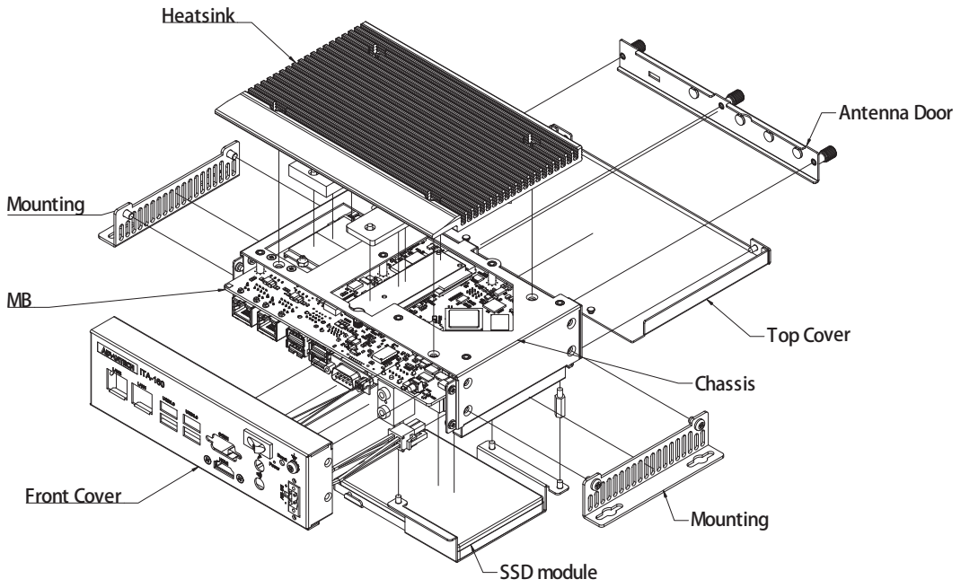
图 1.3: ITA-160 分解图
