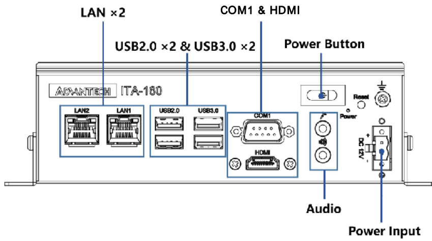
ITA-160 前视图
